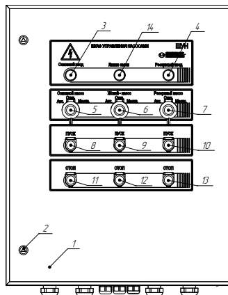
Рисунок 1–Расположение устройств внутри шкафа
